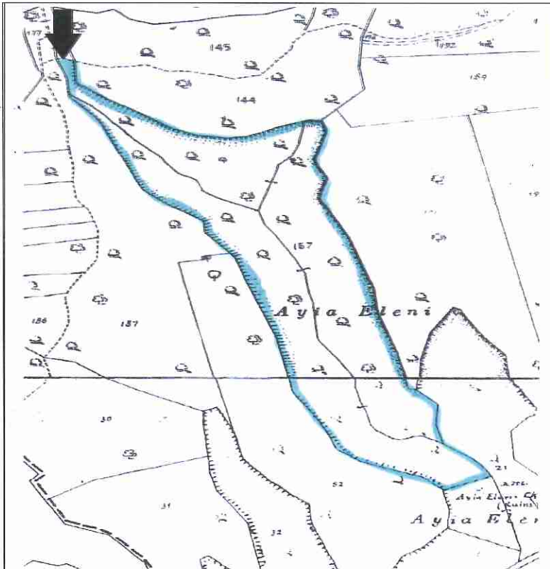
Χωρομετρικό Σχέδιο.
